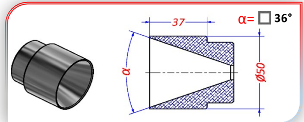
Semi-pressure RS 25 die in steel DS 25
